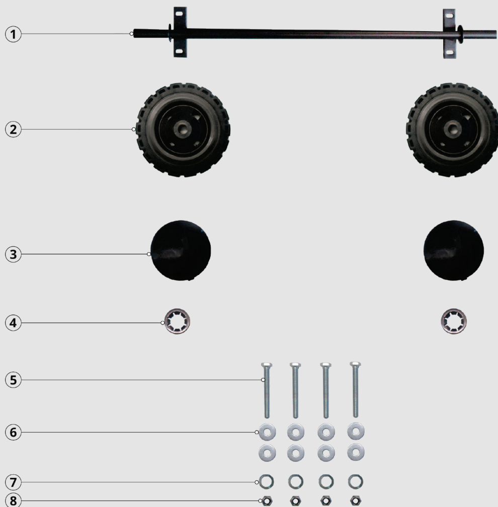
Imagen 20: Lista de materiales del Kit 2: Eje y ruedas.
