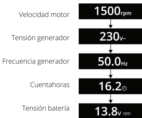
Imagen 11: Parámetros medibles en la placa de control DSE 3110.
