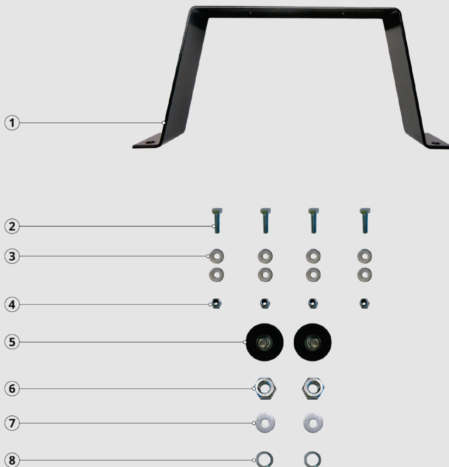
Imagen 21: Lista de materiales del Kit 3: Soporte
