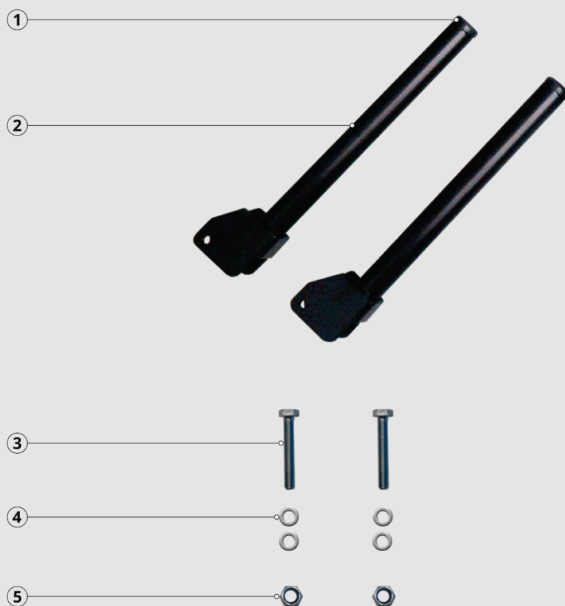
Imagen 19: Lista de materiales del Kit 1: Manerales.
