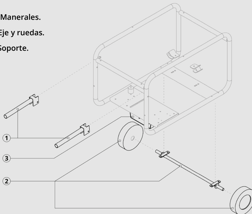
Imagen 18: Componentes del Kit transporte Dagartech
