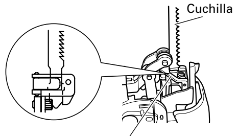
Portacuchilla
