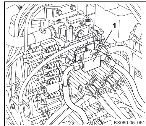
Válvula mecánica de conmutación
