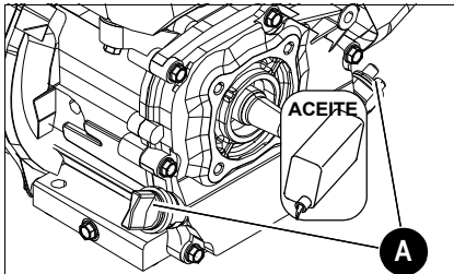
Fig. 77: Rellenar aceite de motor (motor de gasolina)
