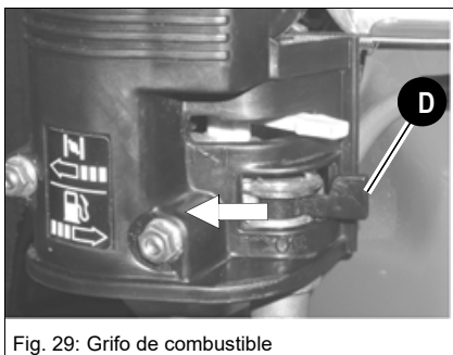
Fig. 29: Grifo de combustible
