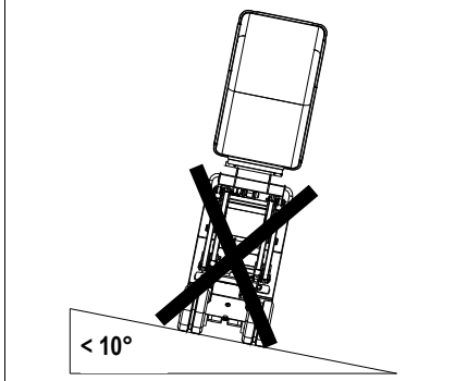
Fig. 42: Desplazamiento en pendientes con la caja del volquete en altura, cargada y sin carga
