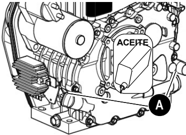
Fig. 77: Rellenar aceite de motor (motor diesel)
