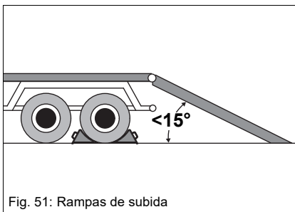
Fig. 51: Rampas de subida
