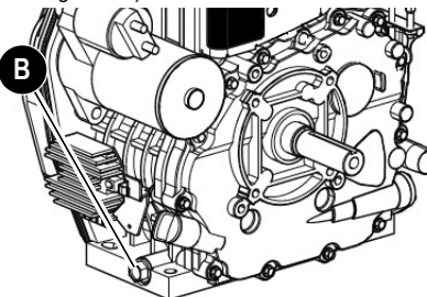
Fig. 78: Vaciar el aceite de motor (motor diesel)
