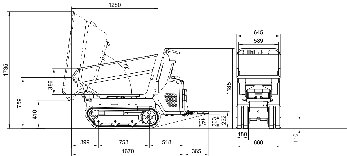
Fig. 95: Dimensiones del vehículo (modelo DT05-D con caja de volquete)
