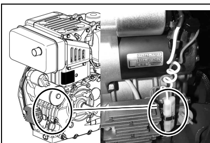
Fig. 94: Fusible motor diésel
