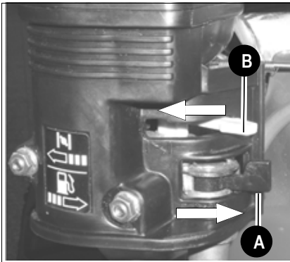
Fig. 22: Grifo de combustible
