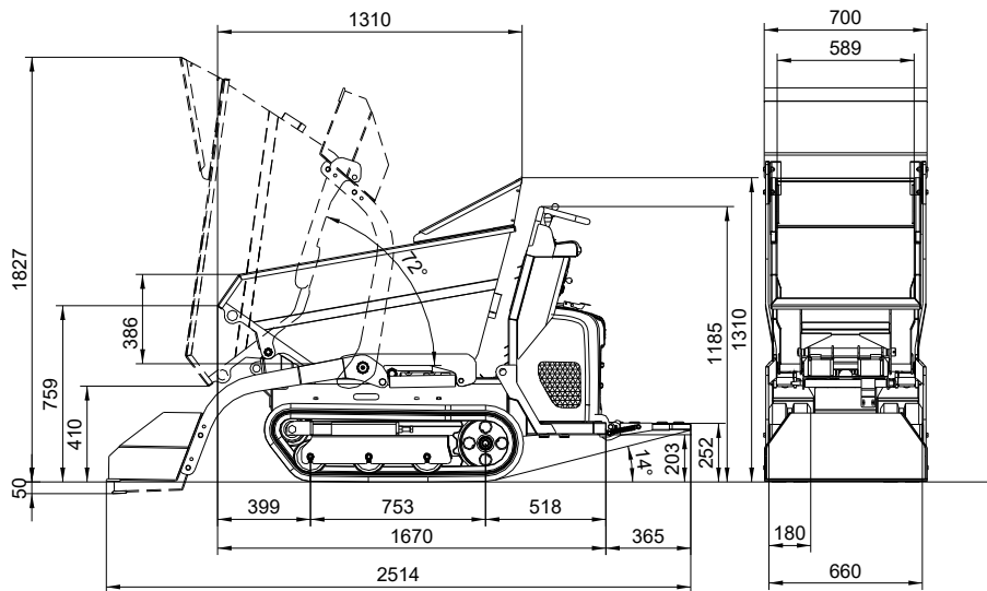
Fig. 96: Dimensiones de la máquina (modelo DT05-D con caja de volquete y dispositivo autocargador)
