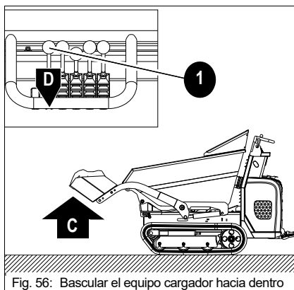
Fig. 56: Bascular el equipo cargador hacia dentro
