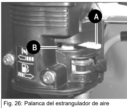
Fig. 26: Palanca del estrangulador de aire
