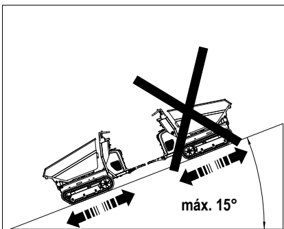
Fig. 41: Conducción en pendiente sin carga
