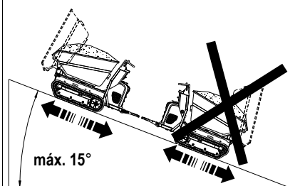
Fig. 41: Conducción en pendiente con carga
