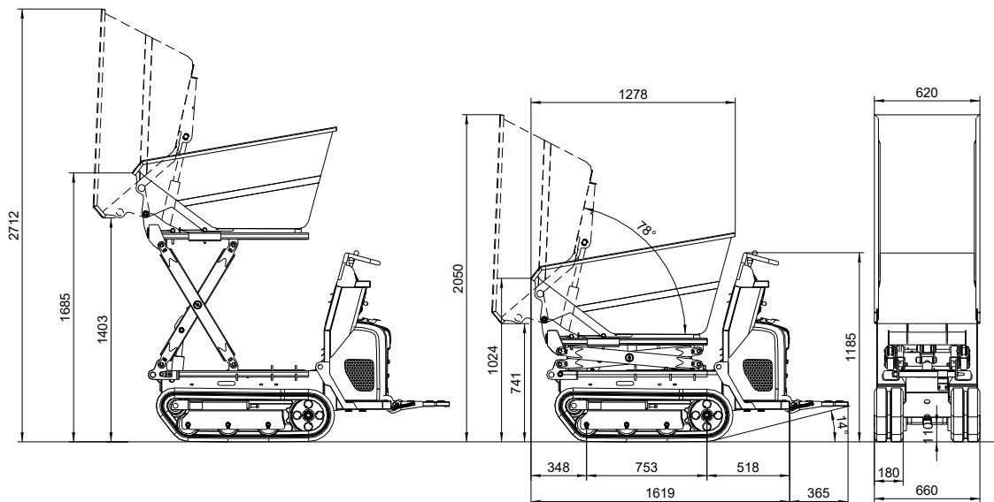
Fig. 98: Dimensiones del vehículo (modelo DT05-D con caja del volquete basculable hacia arriba)
