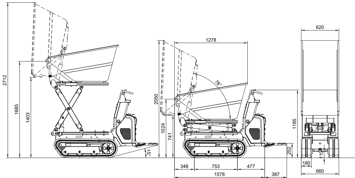
Fig. 102: Dimensiones del vehículo (modelo DT05-P con caja del volquete basculable hacia arriba)
