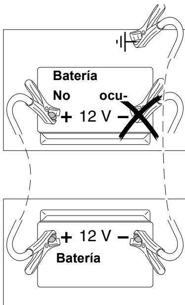
Fig. 38: Ayuda de arranque con cables de arranque
