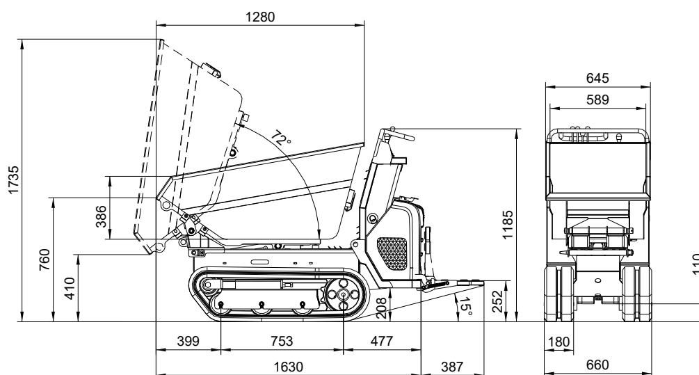
Fig. 99: Dimensiones del vehículo (modelo DT05-P con caja de volquete)
